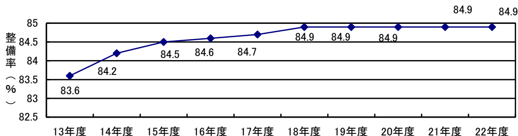
公共下水道整備率の推移
