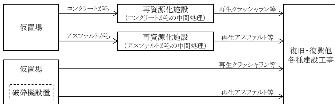
図7 コンクリートがら等の処理フロー
