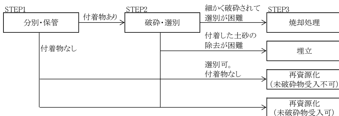
図5 木くずの処理フロー
