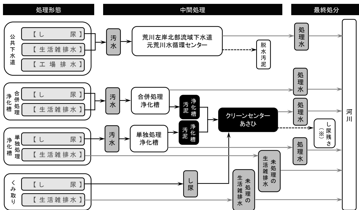
図2-1 生活排水処理の流れ
