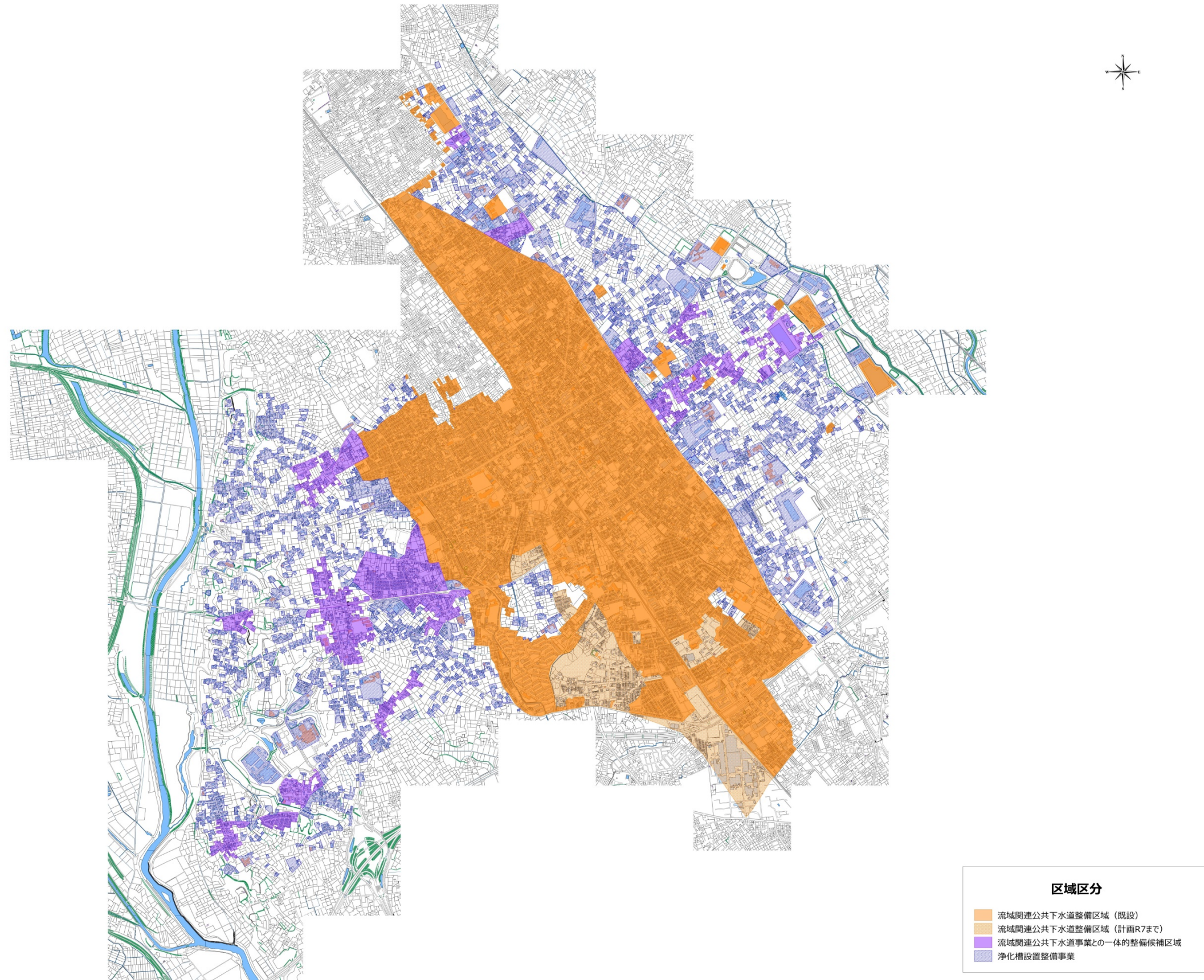
北本市生活排水処理施設整備図
