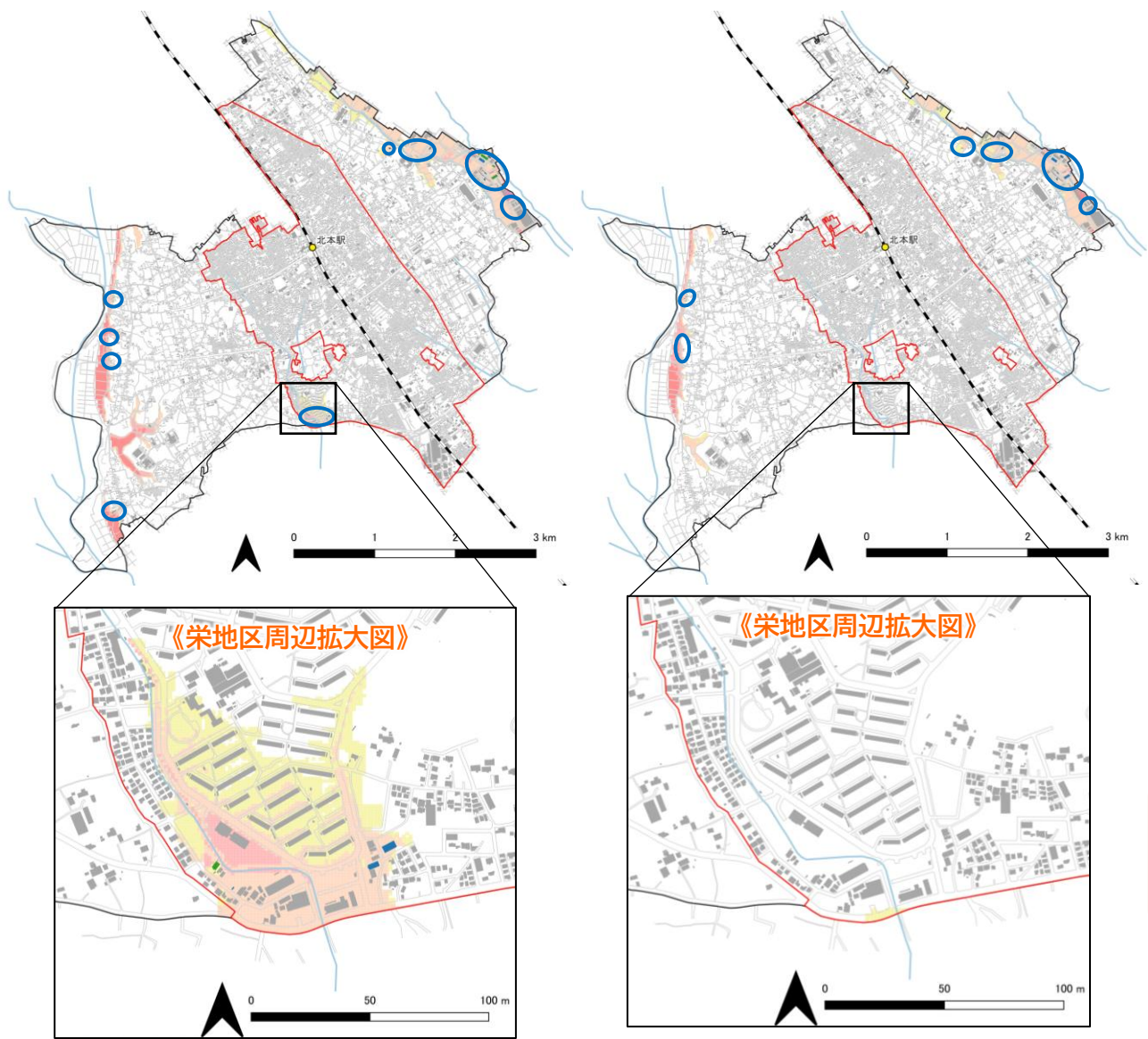
《浸水深（想定最大規模）×建物高さ》
