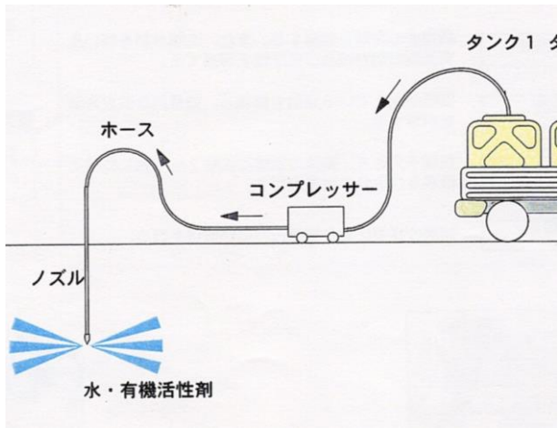
灌注作業概略図
