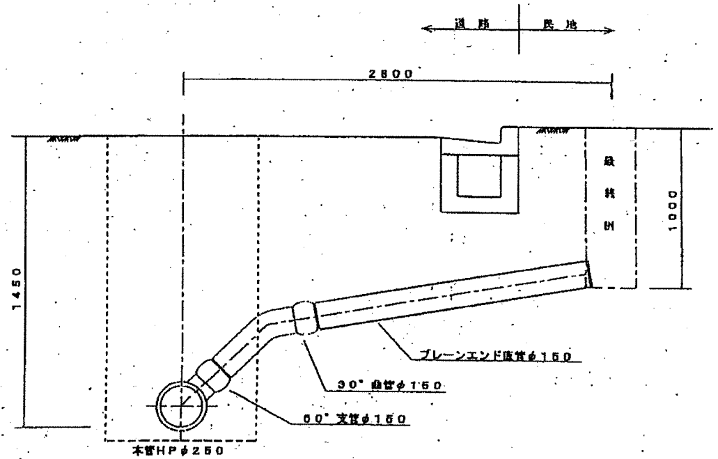
断面図
