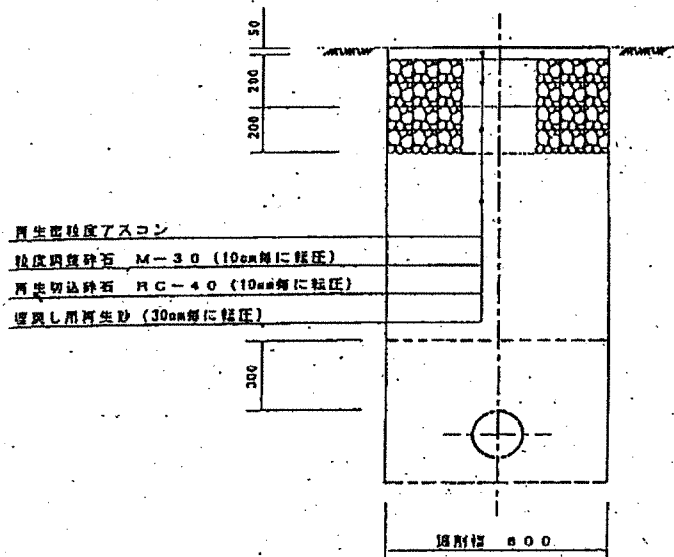
復旧図
